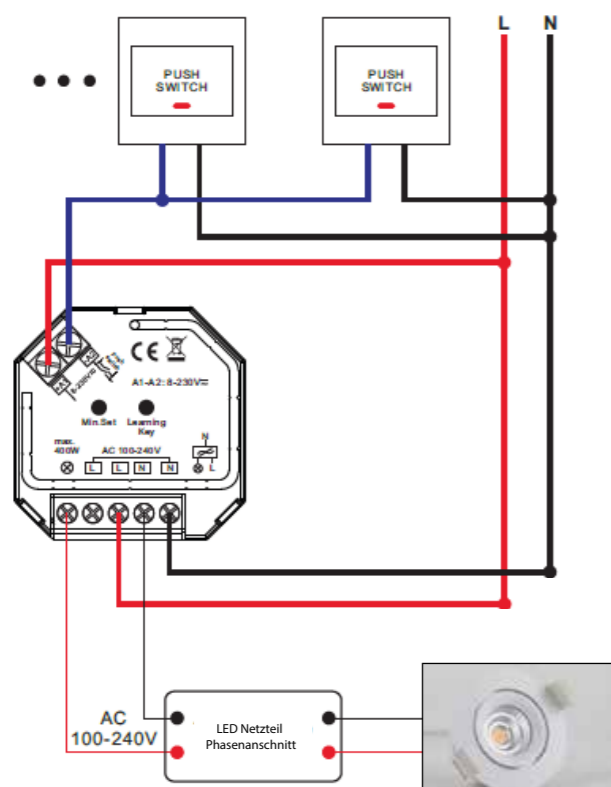
(1)Push-Dimm mit Taster
